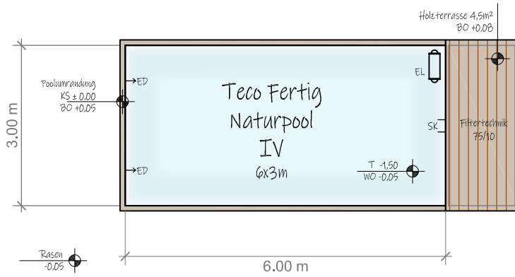
Teco-Fertig-Naturpool mit Poolumrandung (Holz)
